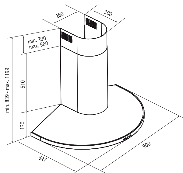
Ausklüngen und Schachtkürzungen nach Skizze
